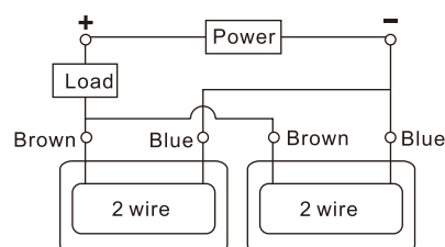
3. PARALELNI PRIKLOP (ALI)
