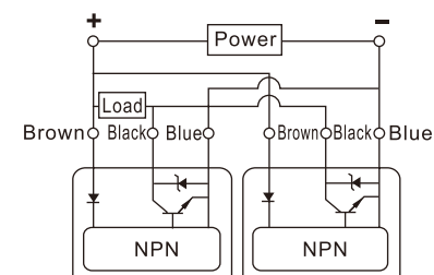
3. PARALELNI PRIKLOP (ALI)
