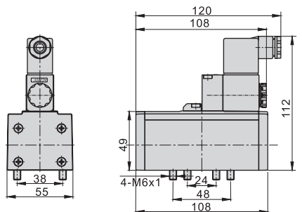
ISO 2 5/2 BCV
