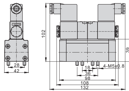
ISO 1 5/3
