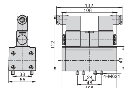
ISO 2 5/2 BCC
