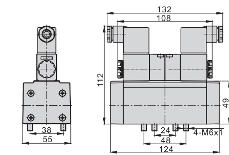
ISO 2 5/3
