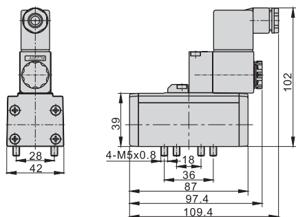
ISO 1 5/2 BCV
